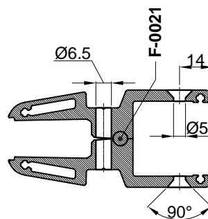
Presjek B-B
