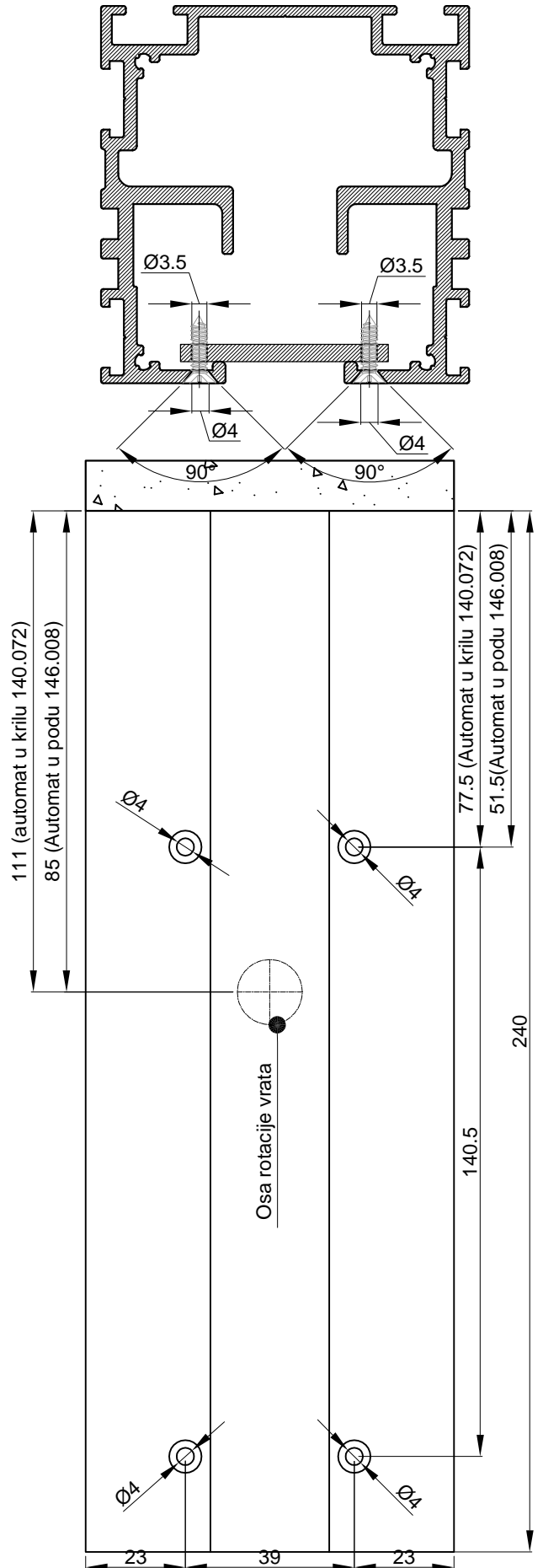
Obrada vodilice i montiranje pločica za prihvat gornjeg okova 146.007
