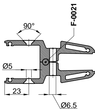
Presjek A-A
