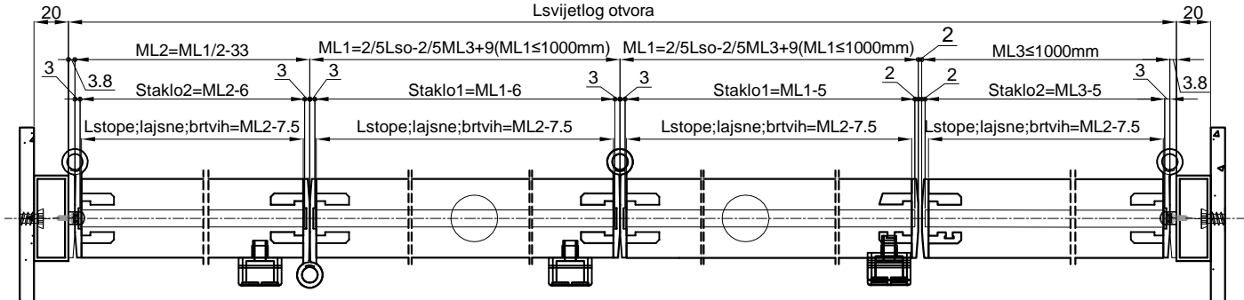
Lsvijetlog otvora
