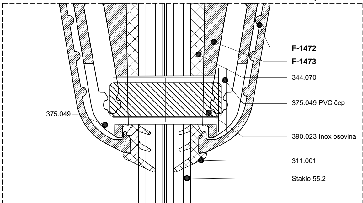
Detalj A
