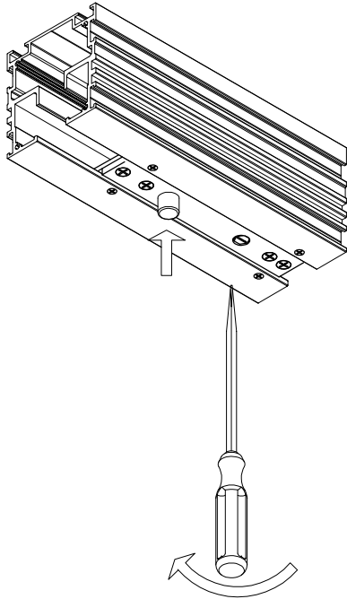
1. Podizanje trna zbog nanošenja vrata
