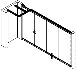
Srednja klizna krila presjek - dolje
