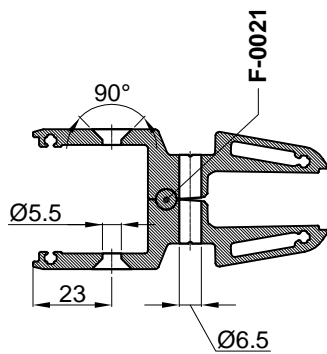
Presjek A-A
