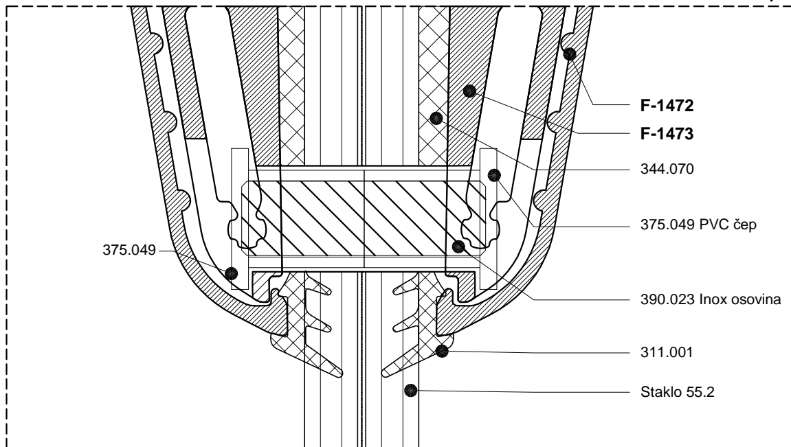
Detalj A
