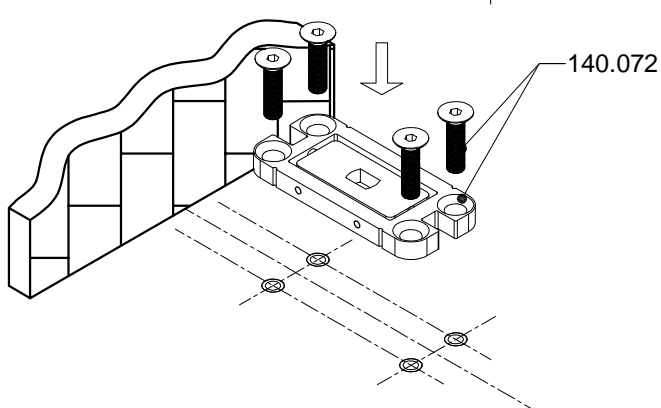
3. Pričvršćivanje pločice vijcima
