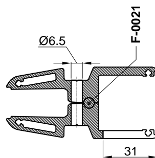
Presjek B-B
