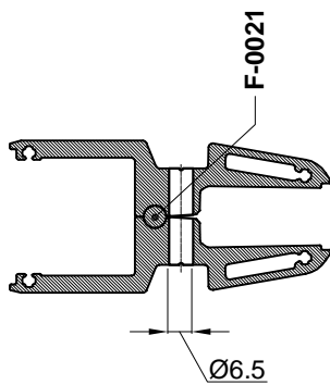
Presjek A-A
