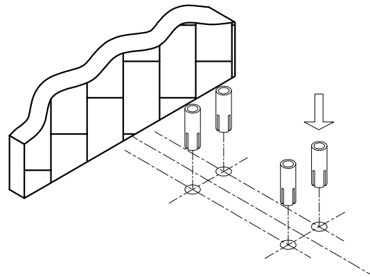
2. Postavljanje čahura za prihvat vijka
