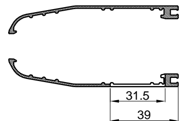
Presjek C-C
