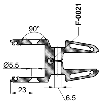
Presjek A-A
