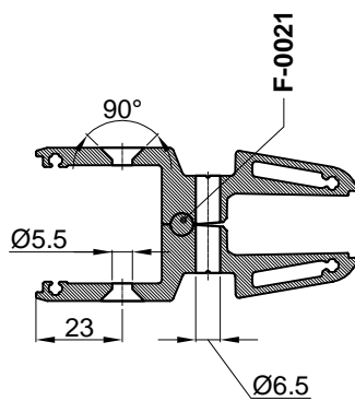
Presjek A-A
